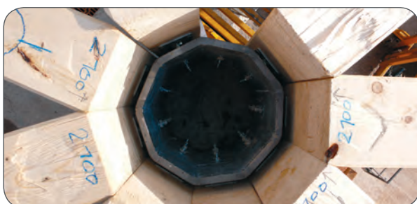
Ein polygonförmiger Stahlrohrabschnitt mit ringsum aufgeschraubten Trägerplatten der RICON® S-Verbinder schließt die Bögen im höchsten Punkt der Kuppel zusammen. Sie wurden einfach rundum eingehängt.
