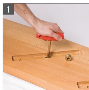
1 Einschraubmutter anschrauben (SW10)
